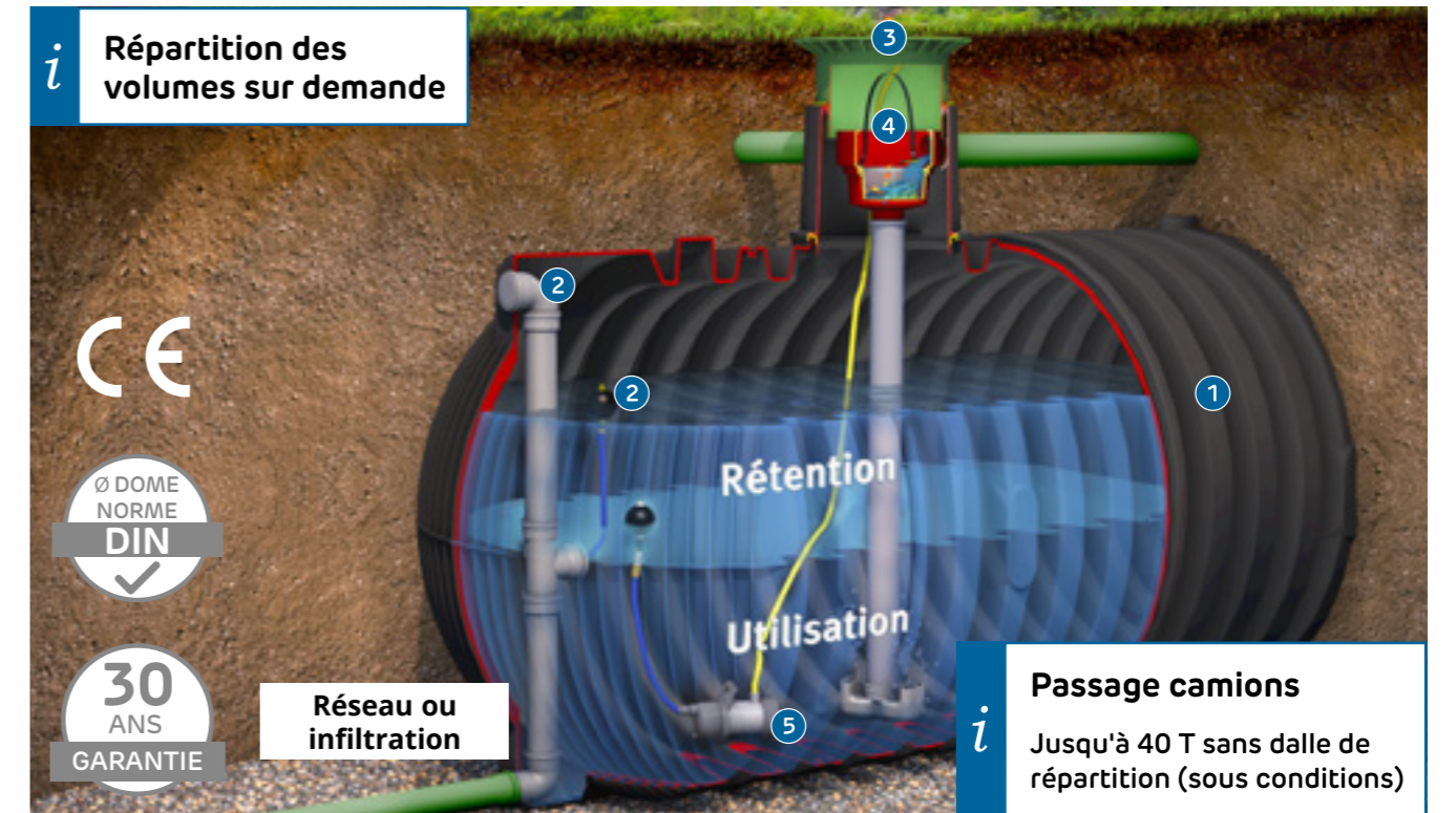
Photo Cuve de rétention Carat XXL Plus avec maxi rehausse, pack filtration et kit technique jardin Confort (accessoires en sus)
