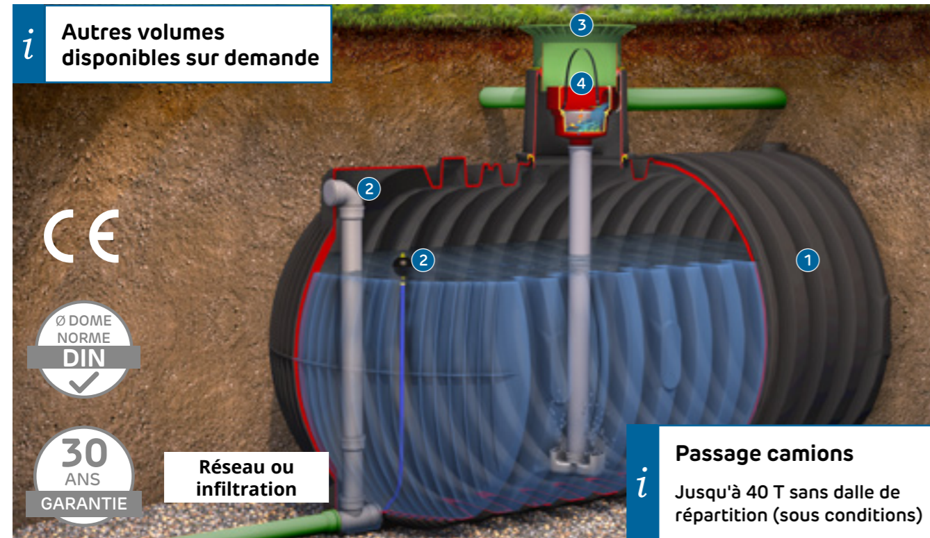
Photo Cuve de rétention Carat XXL avec maxi rehausse et pack filtration (accessoires en sus)
