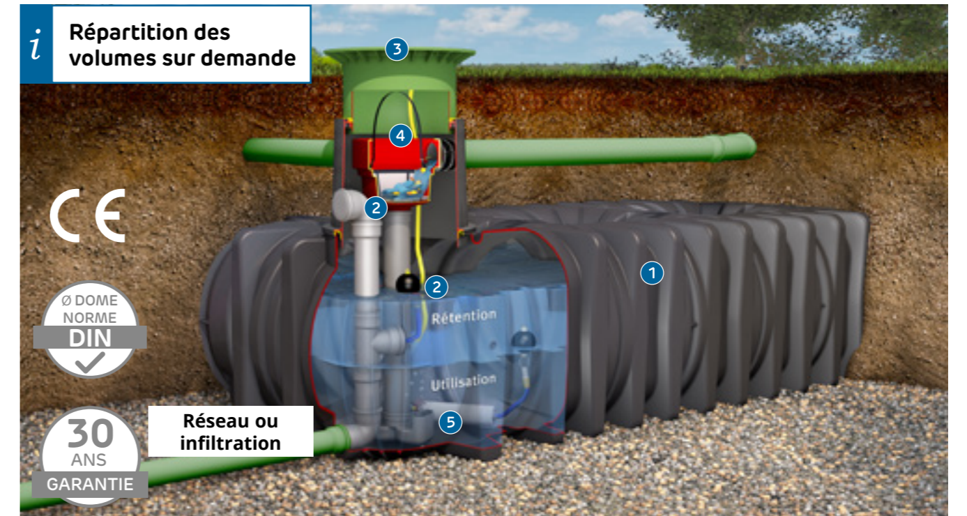
Photo : Cuve de rétention Platine XL/XXL Plus avec maxi rehausse, pack filtration et kit technique jardin Confort (accessoires en sus)
