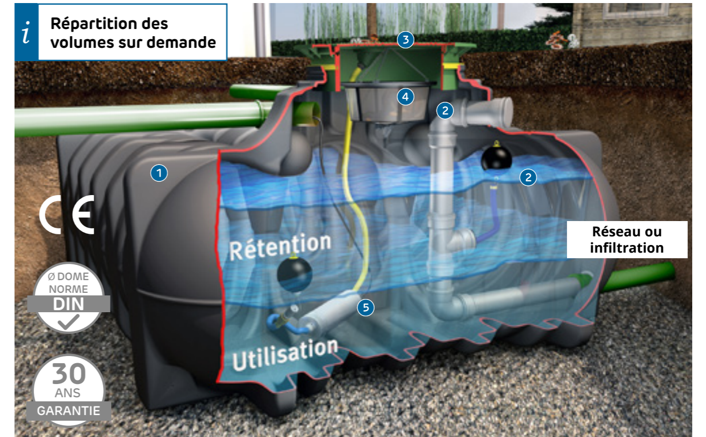
Photo : Cuve de rétention Platine Plus avec mini rehausse, panier filtrant et kit technique jardin Confort (accessoires en sus)
