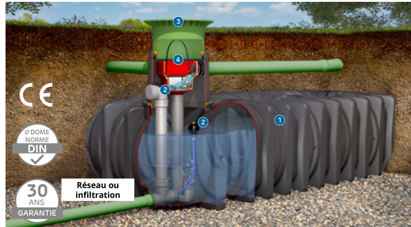
Photo : Cuve de rétention Platine XL/XXL avec maxi rehausse et pack filtration (accessoires en sus)
