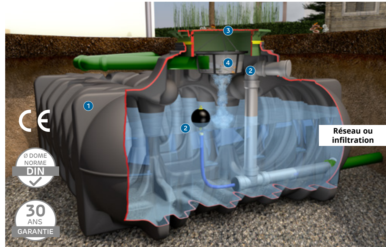
Photo : Cuve de rétention Platine avec mini rehausse et panier filtrant (accessoires en sus)
