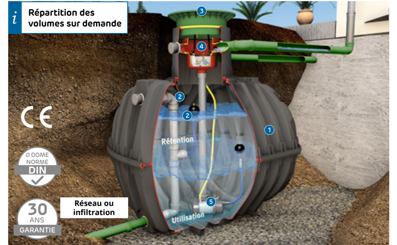
Photo : Cuve de rétention Carat Plus avec mini rehausse, pack filtration et kit technique jardin Confort (accessoires en sus)
