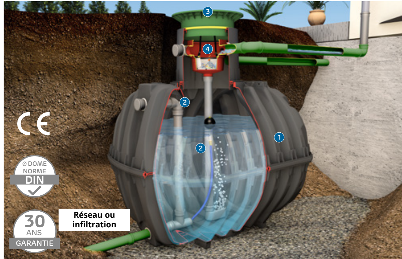
Photo : Cuve de rétention Carat avec mini rehausse et pack filtration (accessoires en sus)
